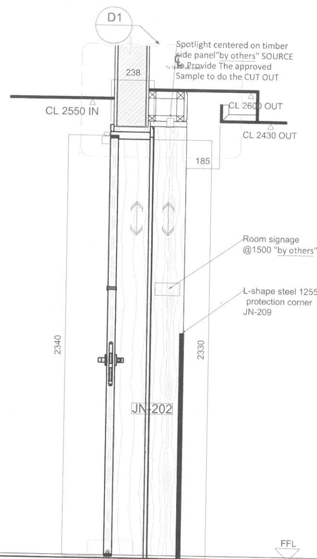
D2 Section
